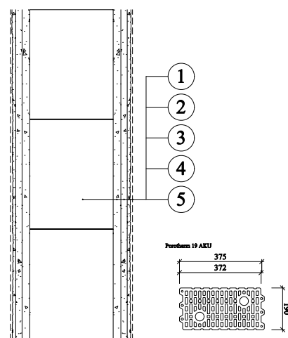
tloušťka zdiva 190 mm
