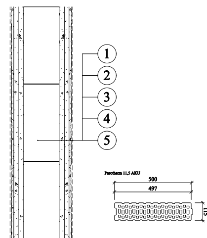
tloušťka zdiva 115 mm
