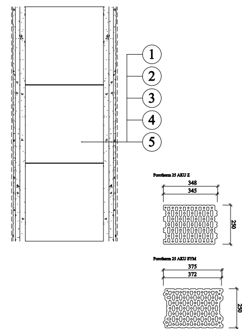
tloušťka zdiva 250 mm
