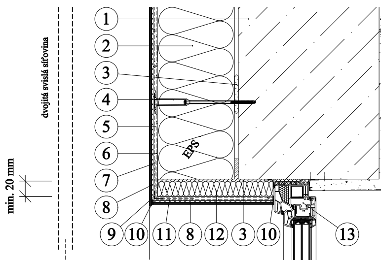
- detail pro nadpraží
