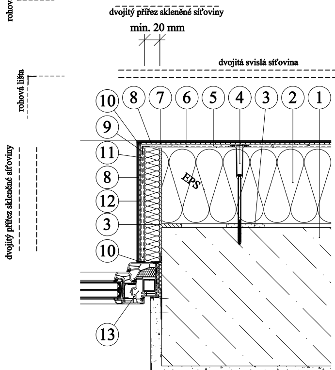
- detail pro ostění
