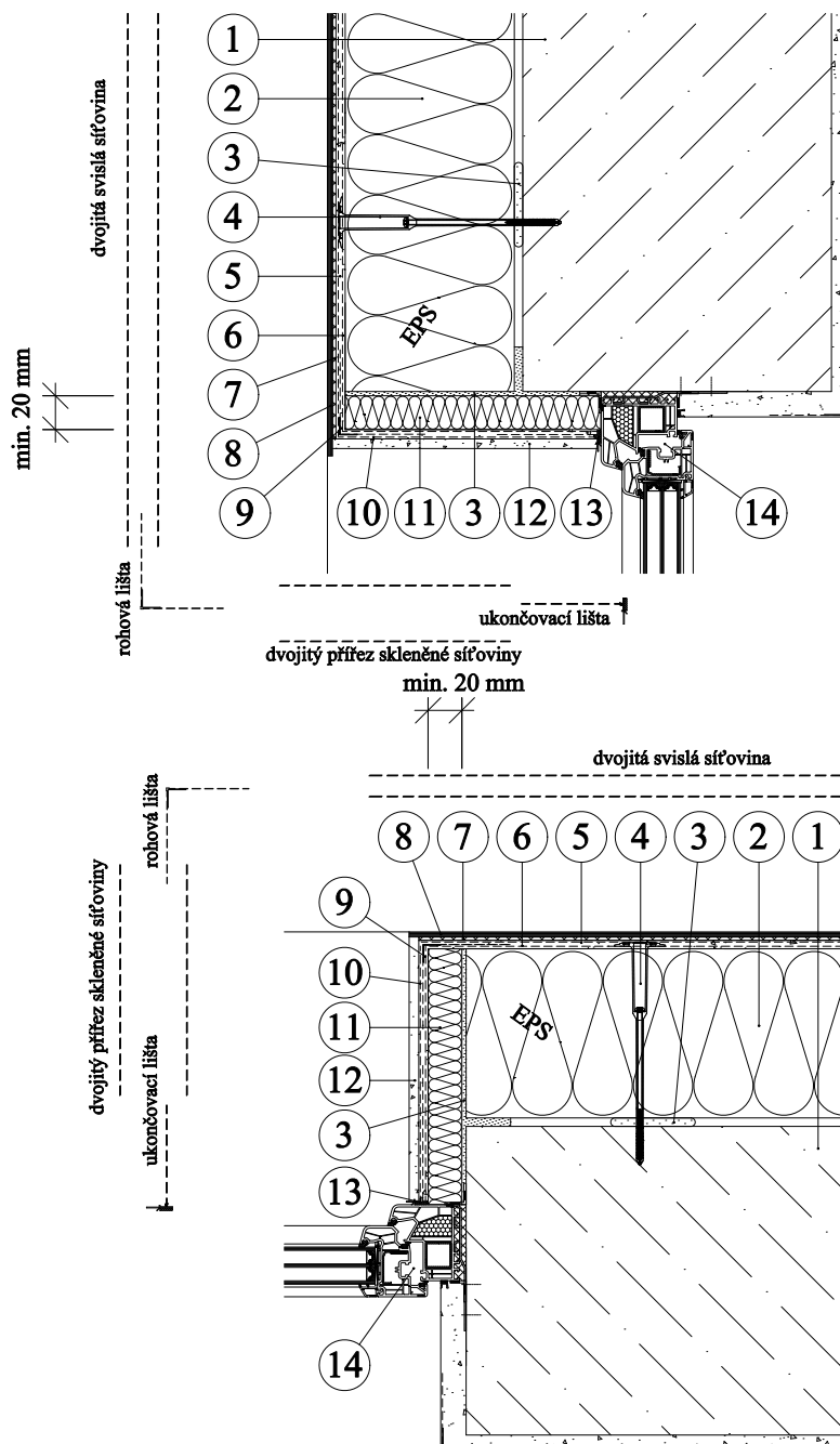
- detail pro nadpraží
