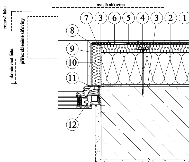
- detail pro ostění
