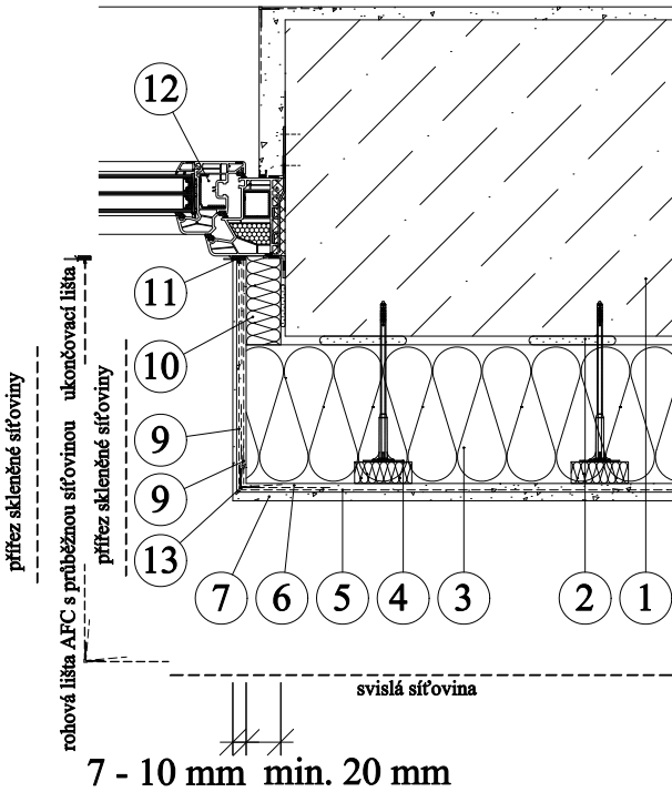
- detail pro ostění
