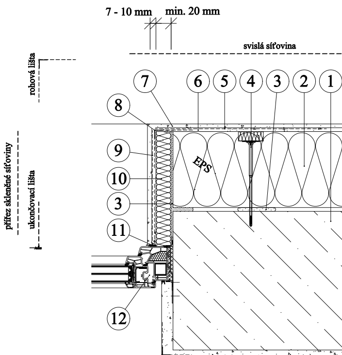
- detail pro ostění
