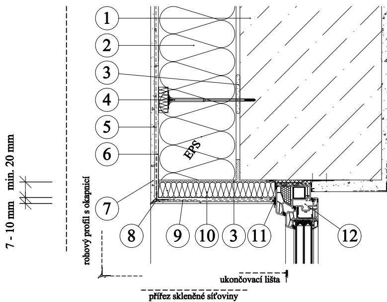
- detail pro nadpraží
