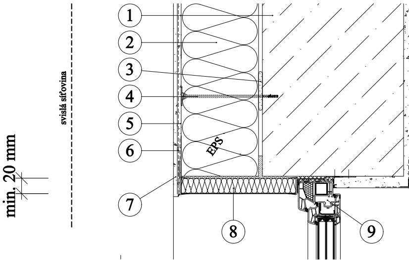
- detail pro nadpraží
