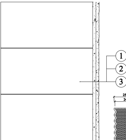
tloušťka zdiva 500 mm
