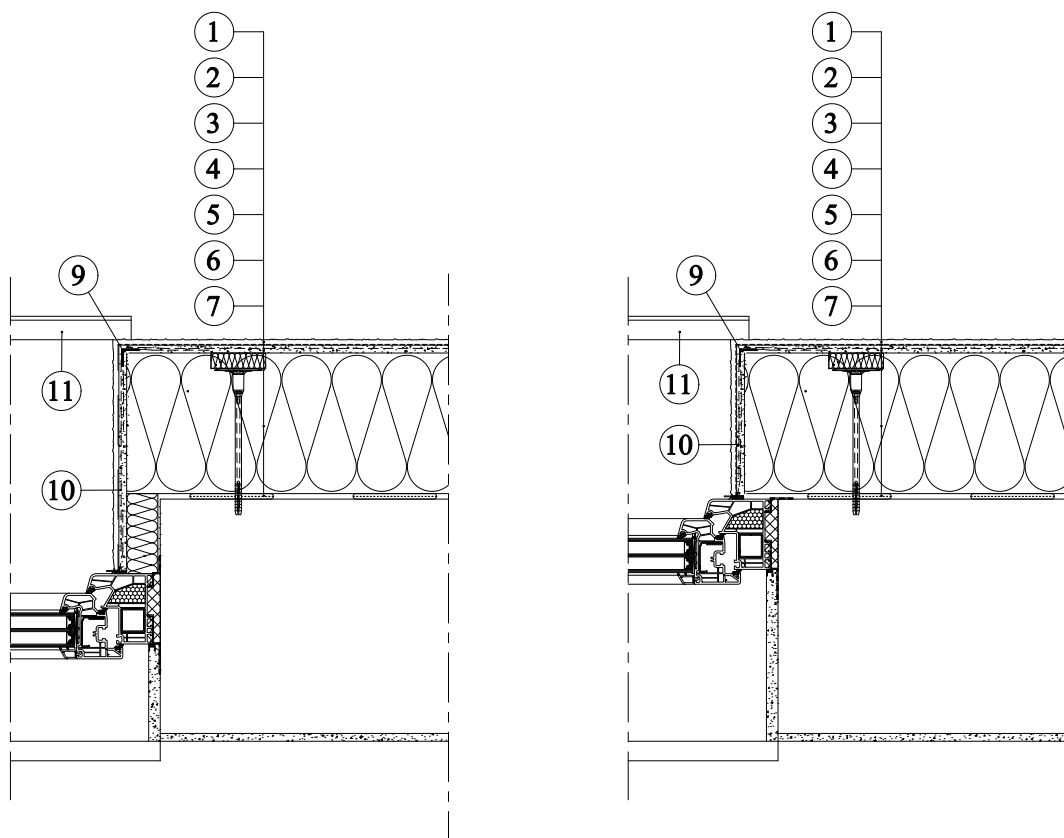
napojení ostění a parapetu
