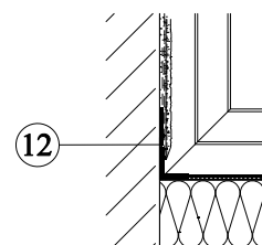
napojení ostění a parapetu
